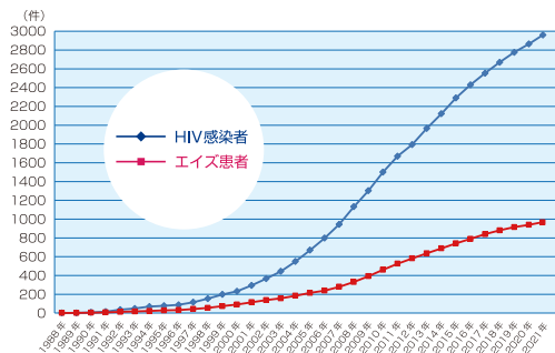
HIV感染者・エイズ患者報告数の年次推移(累計)
