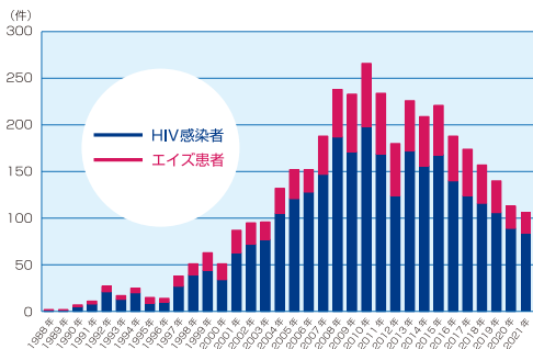
HIV感染者・エイズ患者報告数の年次推移
